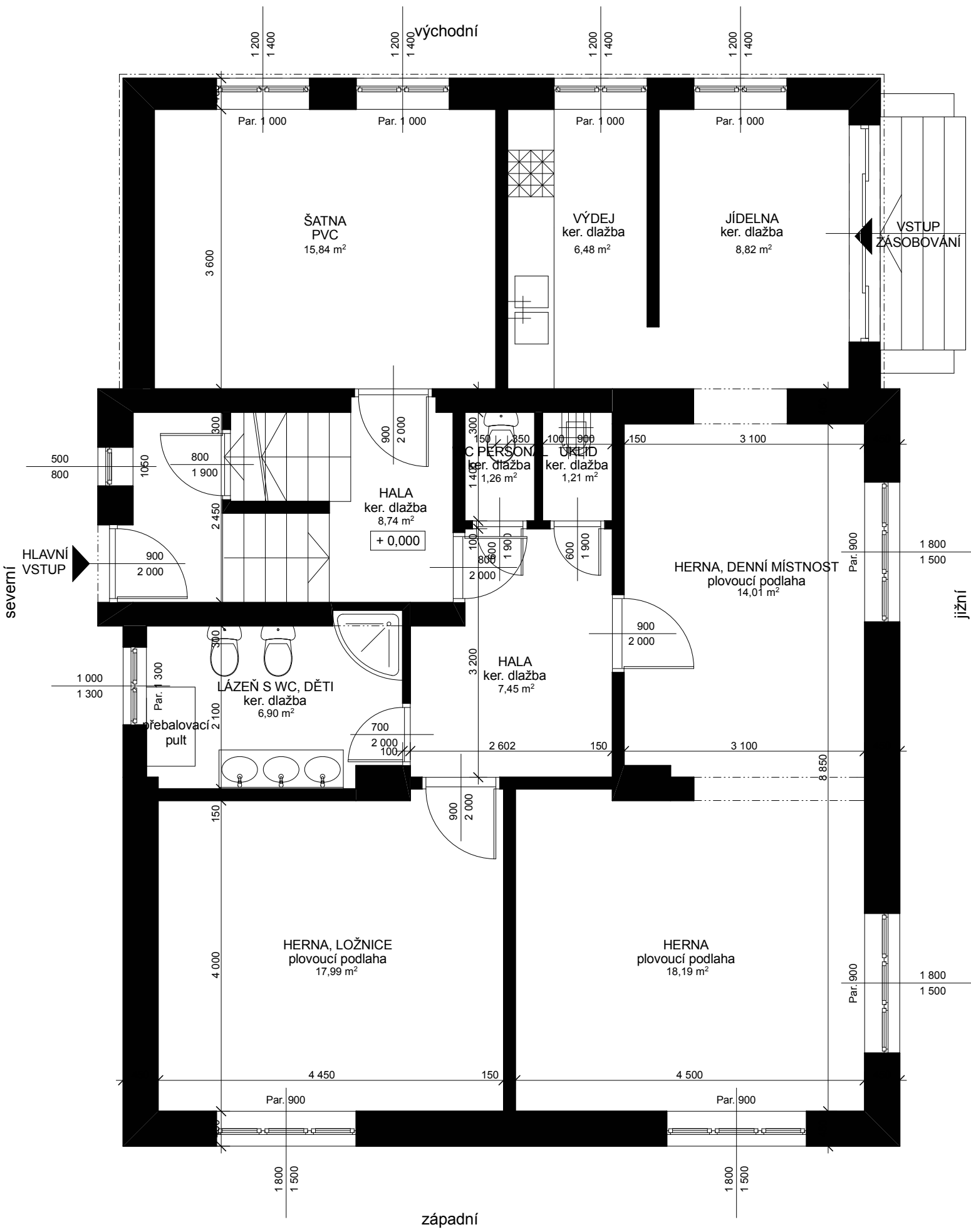
PŮDORYS 1.NP
